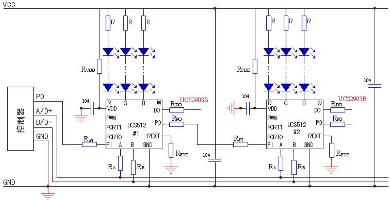
应用图 2: R, G, B 3 字段应用 Application chart2: R, G, B 3 field mode application
