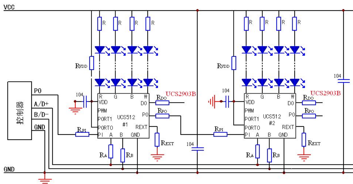
应用图 1: R, G, B, W, 4 字段应用 Application chart 1: R, G, B, W, 4 field mode application
