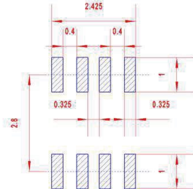
SOT23-8封装脚位尺寸参考图：
